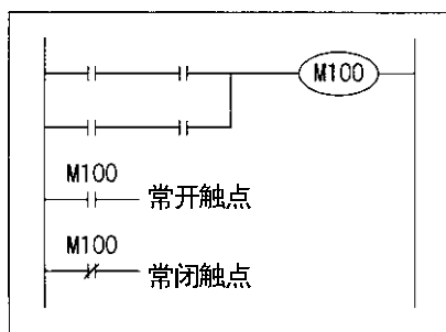
辅助继电器回路
