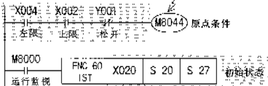
《各个操作》 没有各个模式时，不需要该程序。
