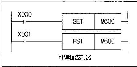
停电保持回路(位置复位方式)
