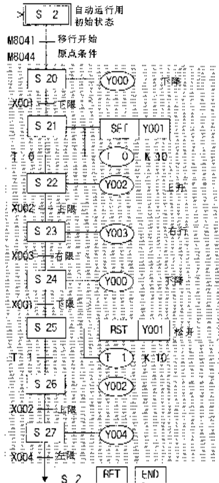
《自动运行》(单步/循环一次/连续)
