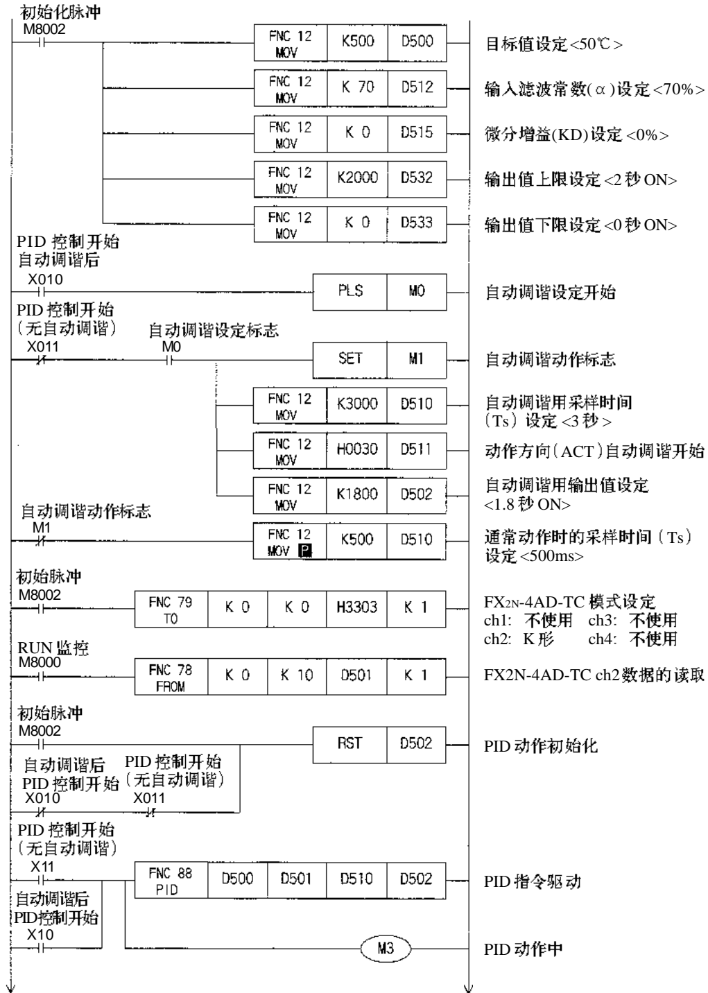
自动调谐+PID控制的程序
