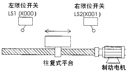
停电保持回路(位置复位方式)
