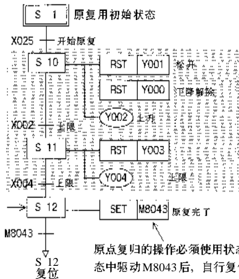
《原点复归》 没有原复模式时，不需要该程序。但在自动运行前需要复位一次 M8043 (原复完毕)。
